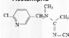
Acetamiprid
