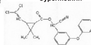
Cypermethrin
