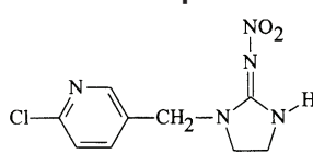
Imidacloprid
