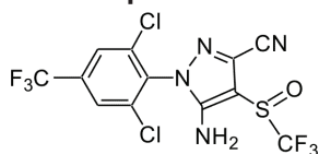
Fipronil
