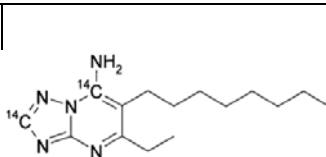
Ametoctradin
