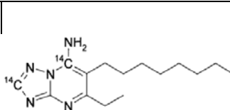
Ametoctradin
